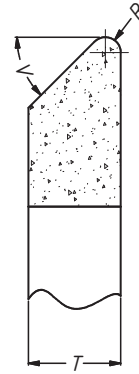
Randform DZ Angabe: T - R - V°
