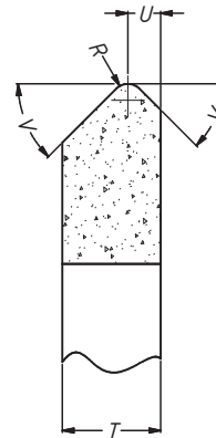
Randform IZ Angabe: T - R - V° - U
