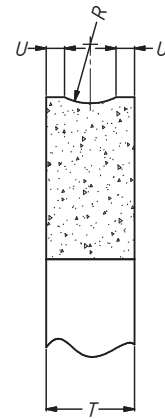
Randform JZ Angabe: T - R - U
