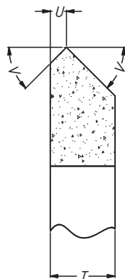
Randform NZ Angabe: T - V° - U
