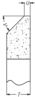
Randform CZ Angabe: T - U - V°
